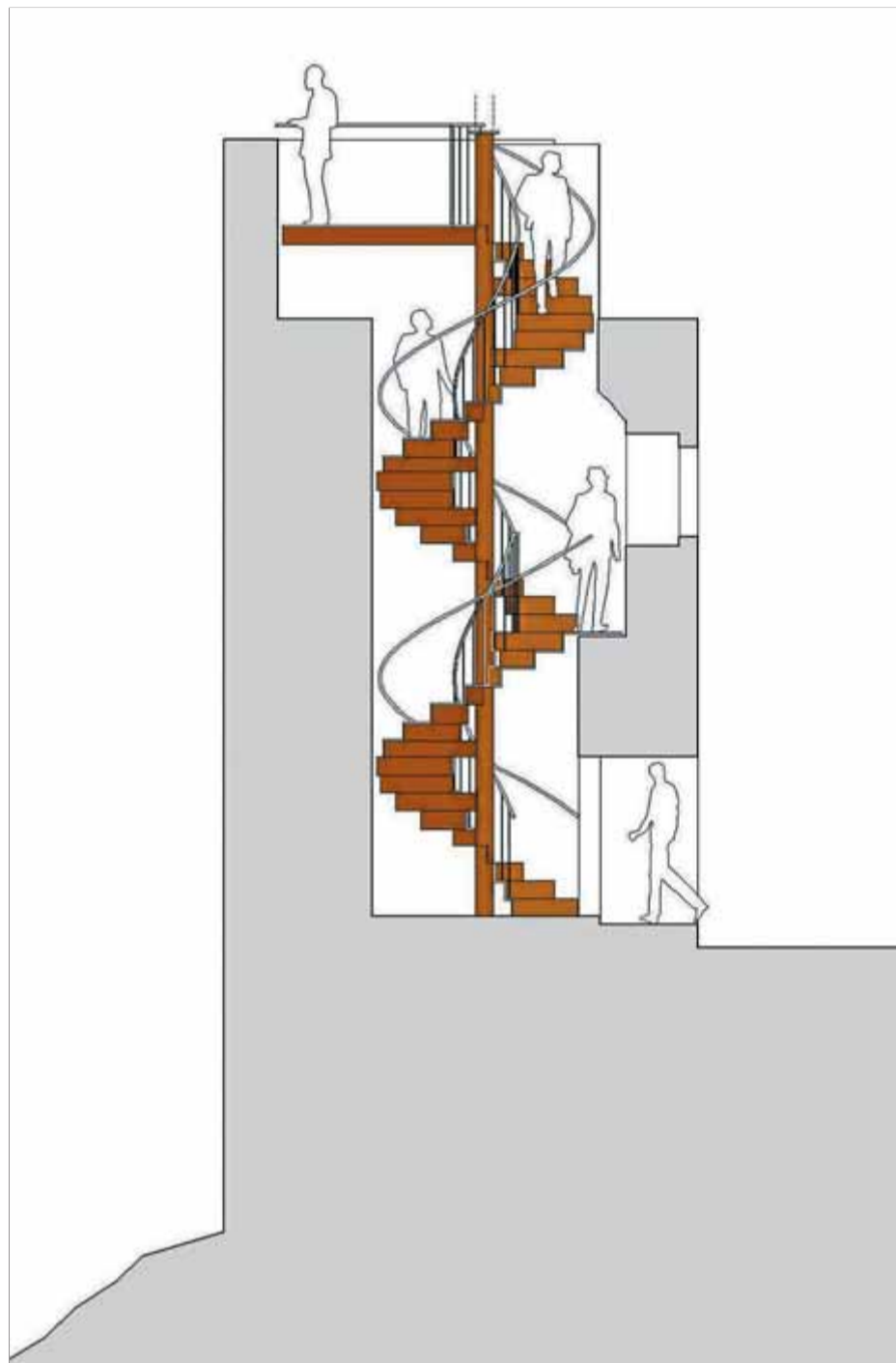
Un dels plànols en què es mostra com quedarà l'interior de la torre ■ AJUNTAMENT LLAGOSTERA
