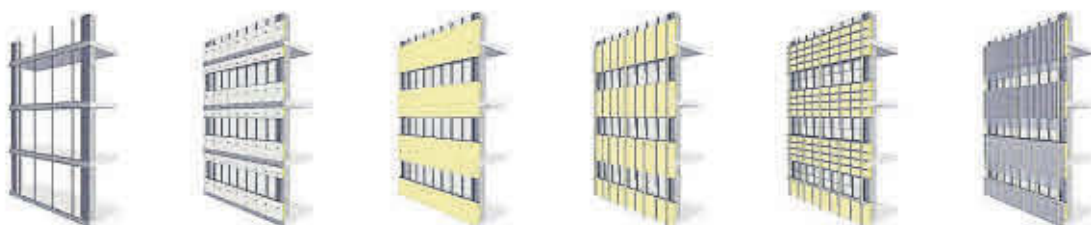
Diferents fases del muntatge de la façana ventilada, segons esquema de Ciprés Group.
